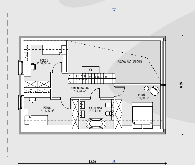
BUDYNEK MIESZKALNY, RZUT PODDASZA
