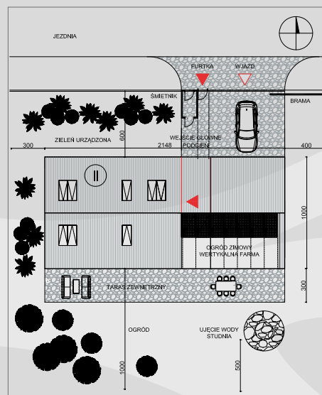
ZAGOSPODAROWANIE TERENU DZIAŁKI
