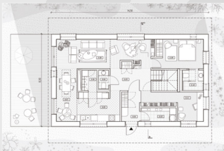
RZUT PARTERU
