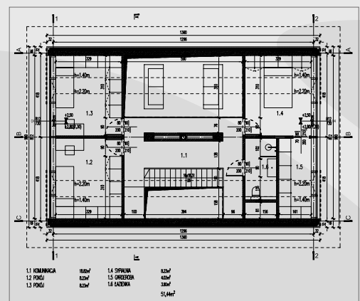
RZUT PODDASZA
