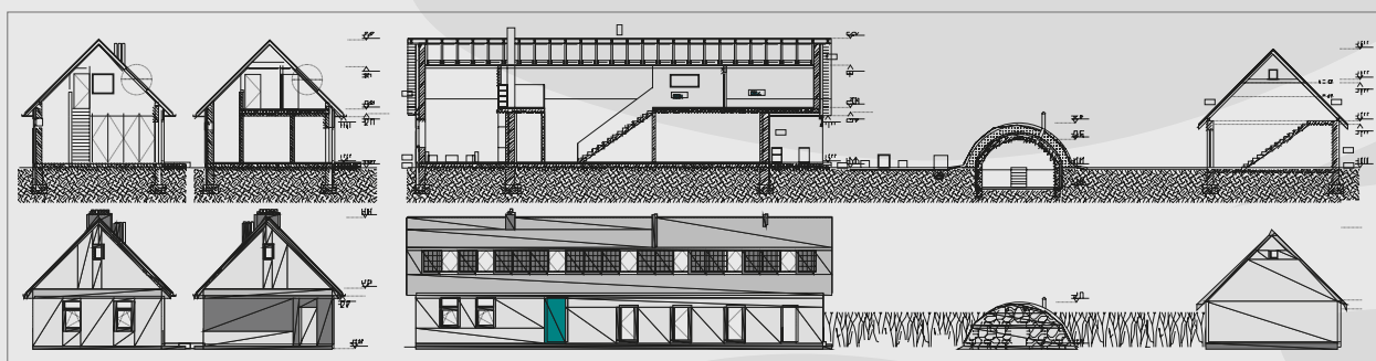
ELEWACJE I PRZEKROJE
