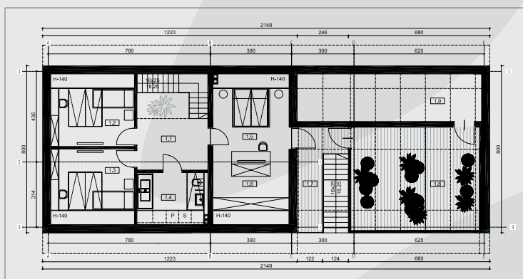
RZUT PIĘTRA
