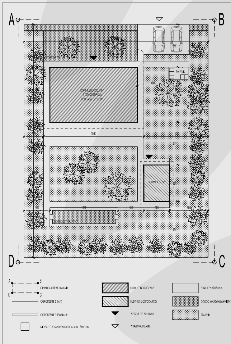
KONCEPCJA ZAGOSPODAROWANIA TERENU
