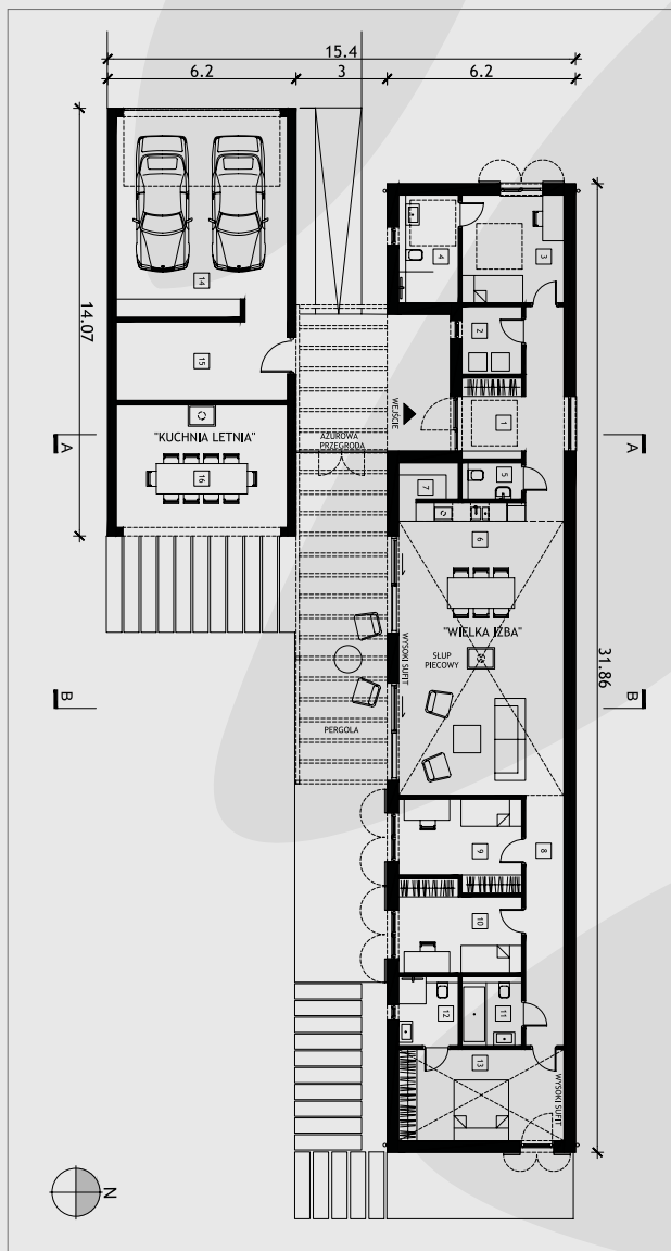
RZUT BUDYNKU MIESZKALNEGO Z GARAŻEM I LETNIĄ KUCHNIĄ | OPIS RZUTU
