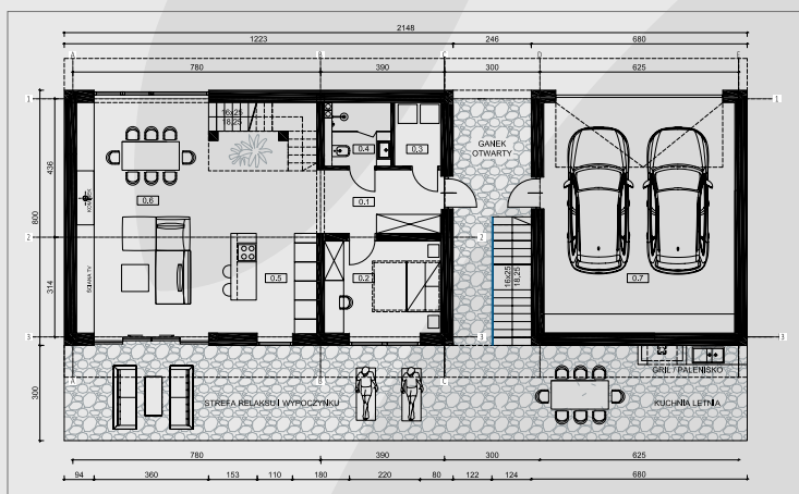
RZUT PARTERU
