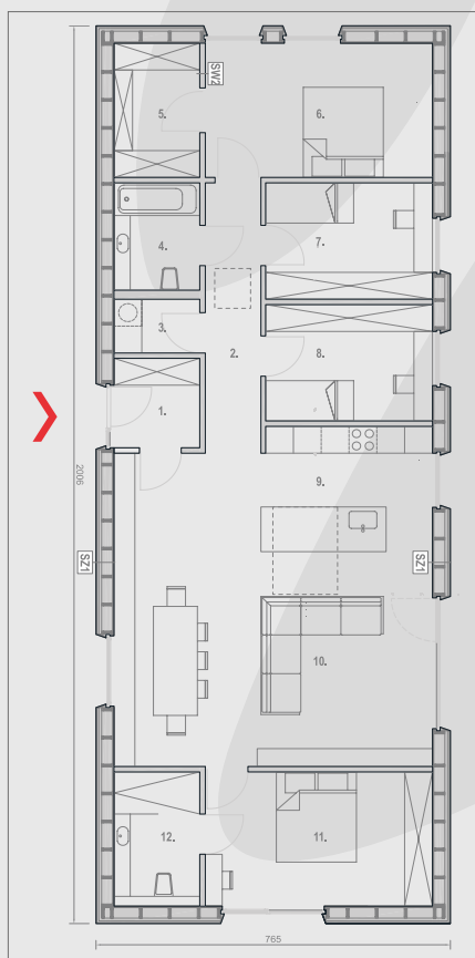
RZUT BUDYNKU MIESZKALNEGO
