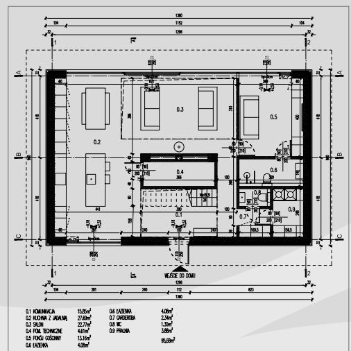
RZUT PARTERU
