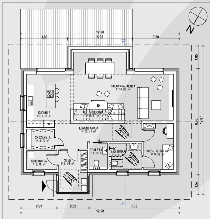
BUDYNEK MIESZKALNY, RZUT PARTERU
