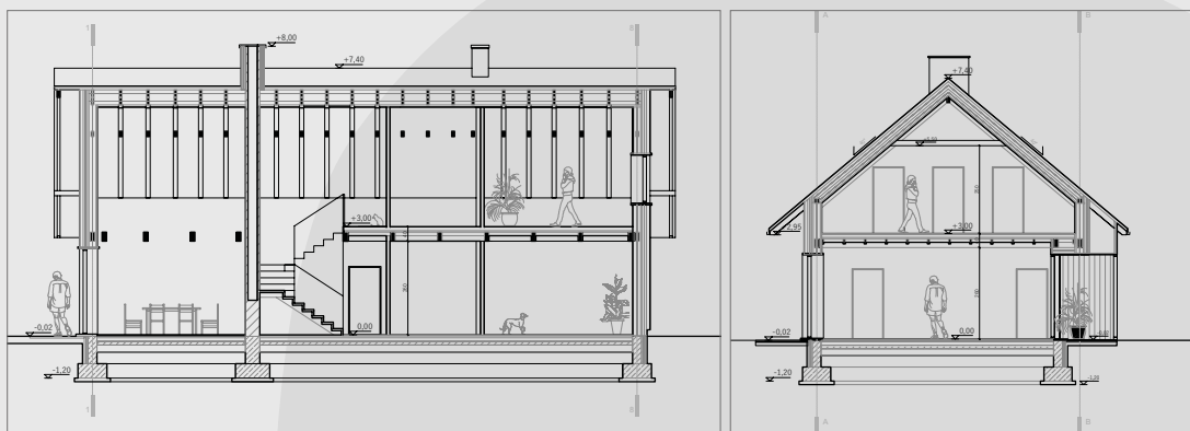
PRZĘCZÓJ B-B,
